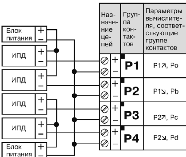
Рисунок В.2 – Схема подключения к вычислителю ИПД
