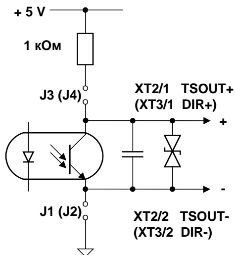
Рис.В.1. Схема окончного каскада универсальных выходов.
