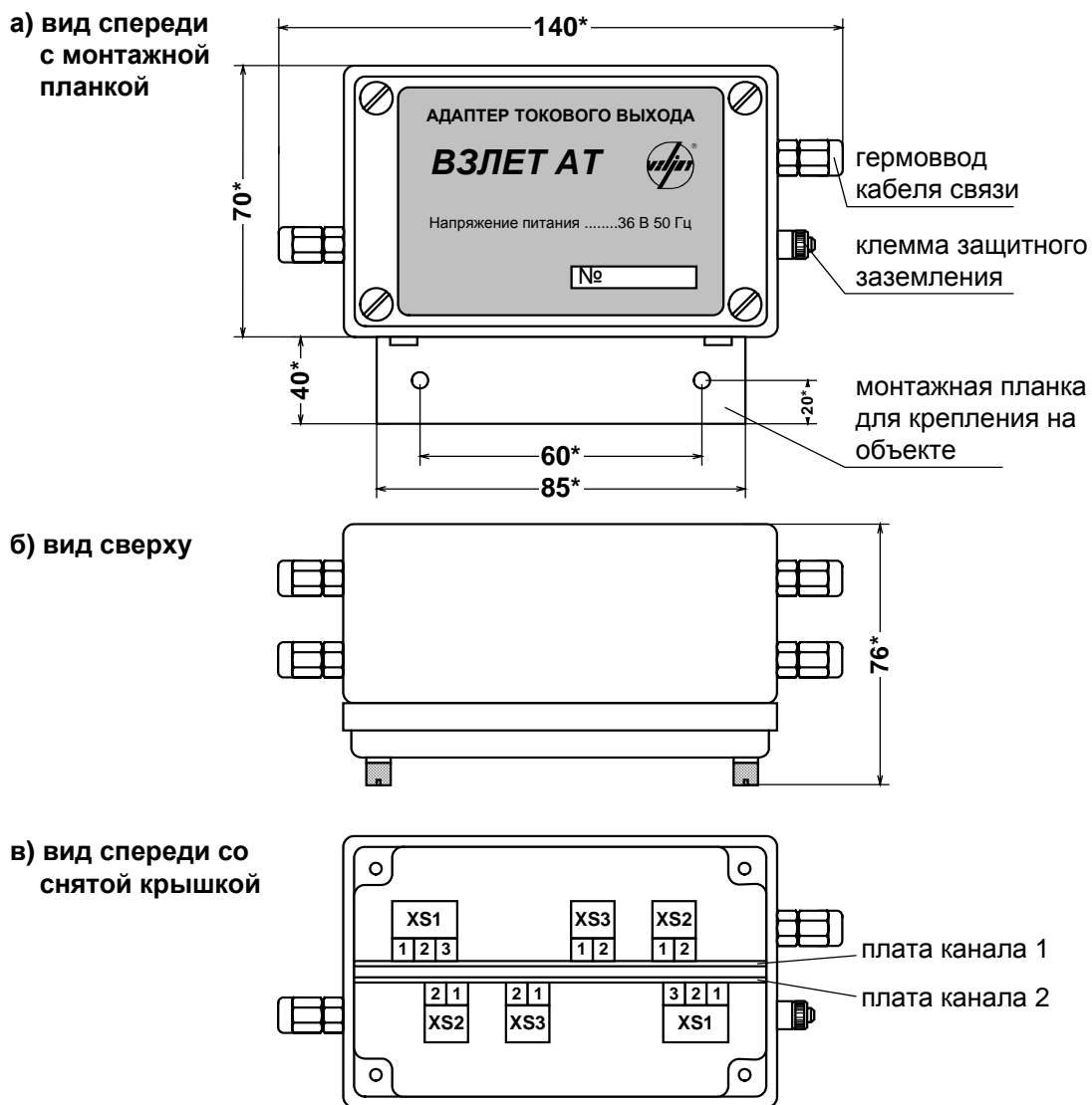
Рис.Г.1. Вид адаптера токового выхода.
