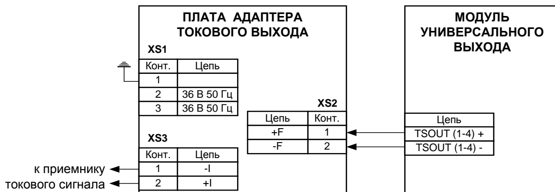
Рис.Г.2. Схема подключения платы адаптера.
