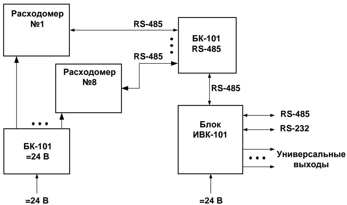
Рис.7. Система сбора данных и выносной индикации на базе комплекса «ВЗЛЕТ ИVK» с использованием BK-101 для 2-8 расходомеров.
