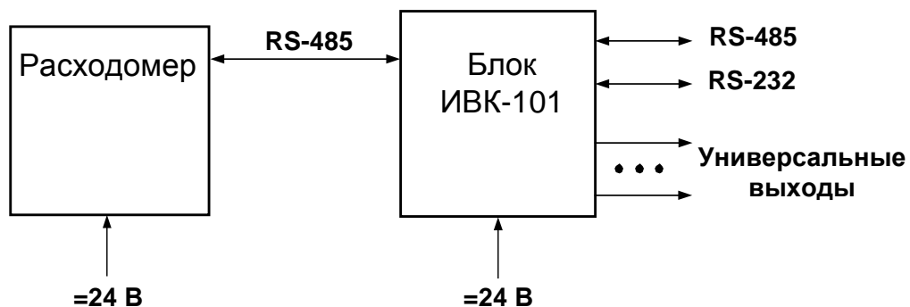
Рис.5. Система сбора данных и выносной индикации на базе комплекса «ВЗЛЕТ ИВК» для одного расходомера.
