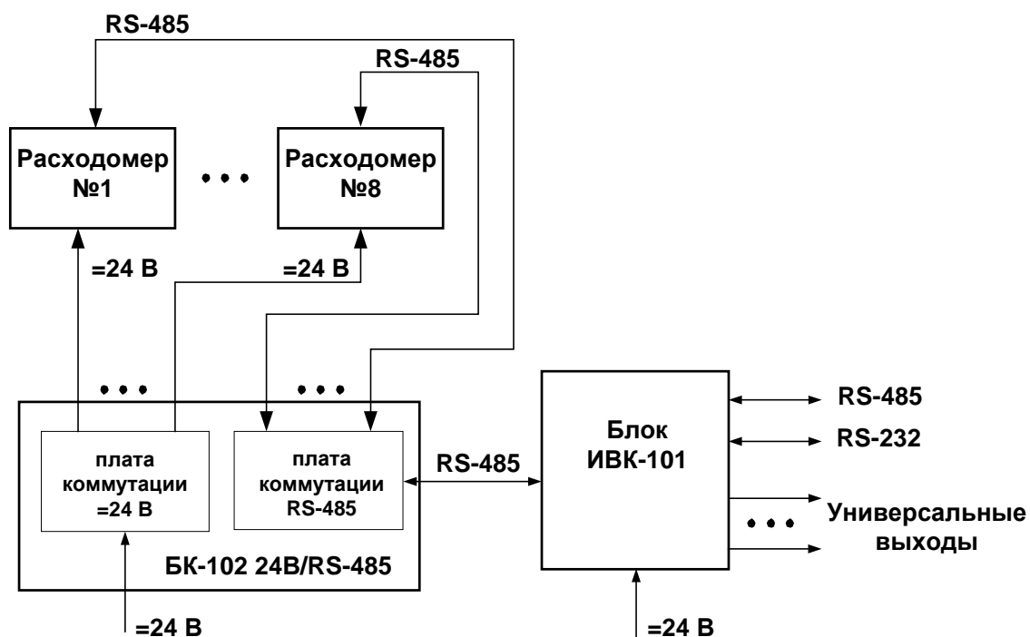
Рис.6. Система сбора данных и выносной индикации на базе комплекса «ВЗЛЕТ ИВК» с использованием БК-102 для 2-8 расходомеров.
